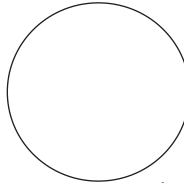
Planet
